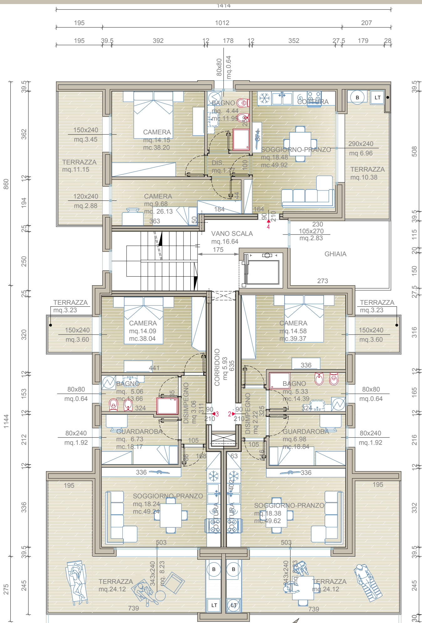
PIANTA PIANO 1°
